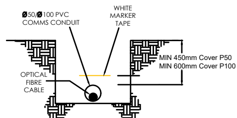
SECTION A-A TRENCH
